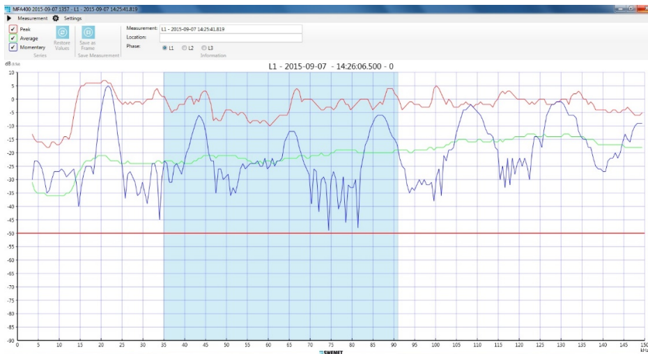
Bild 2 visar mätning i transformatorstationen ca 150 Tv:n
